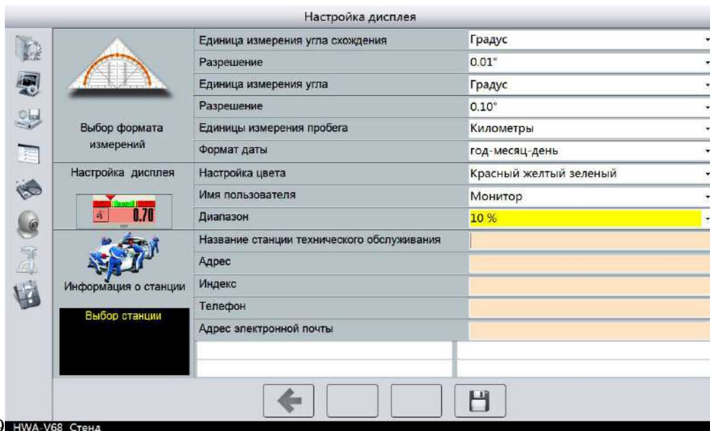
Рис. 39 HWA-V68 Стенд
